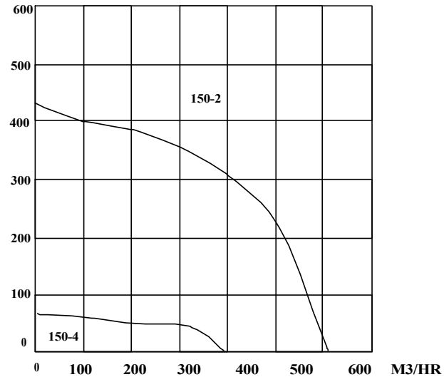
AC-QCFR 150 FAN CURVES
